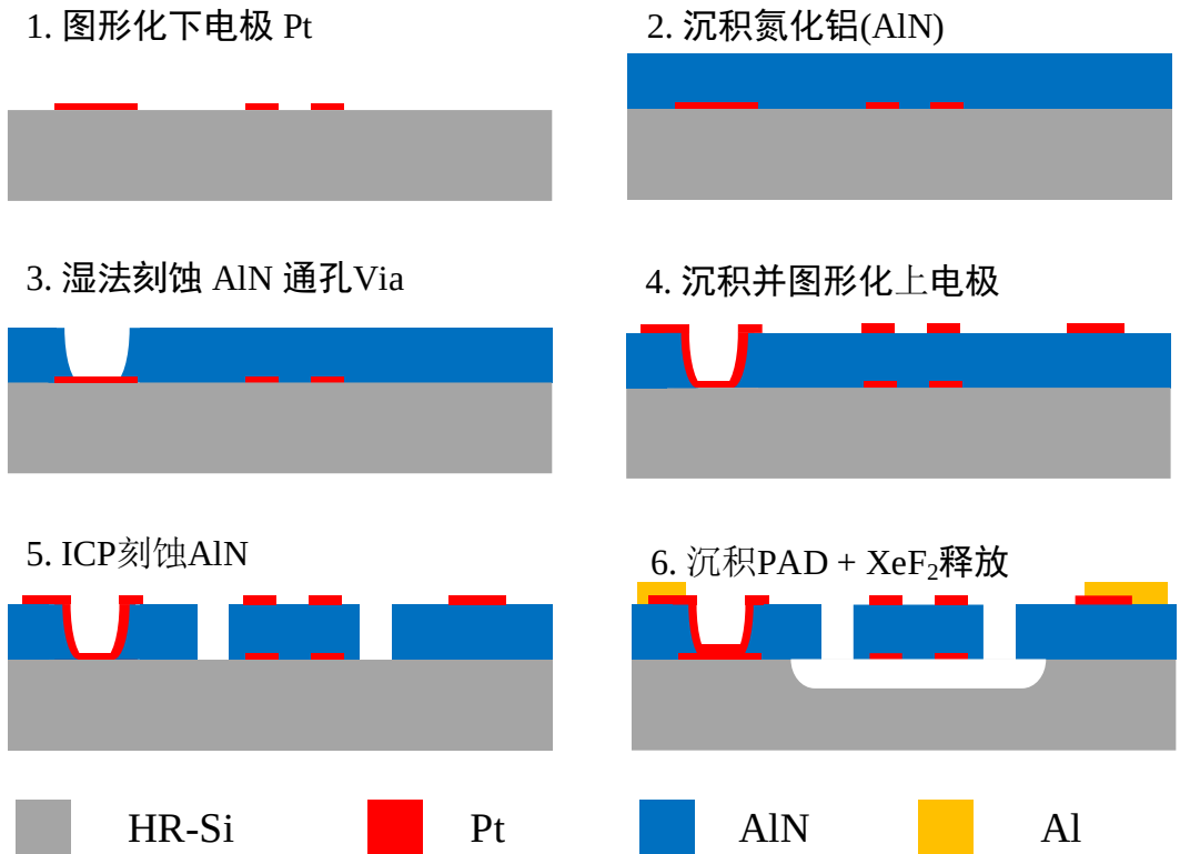
a) 标准工艺流程;
