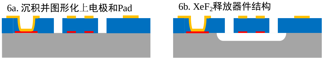
b) 直接使用 PAD#5 (200 nm Al) 作为 上电极和布线 (注: 工艺流程无变化, 只是跳过 GDS#3);
